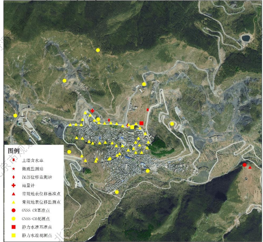
秋林铺村采空区仪器点位分布图
