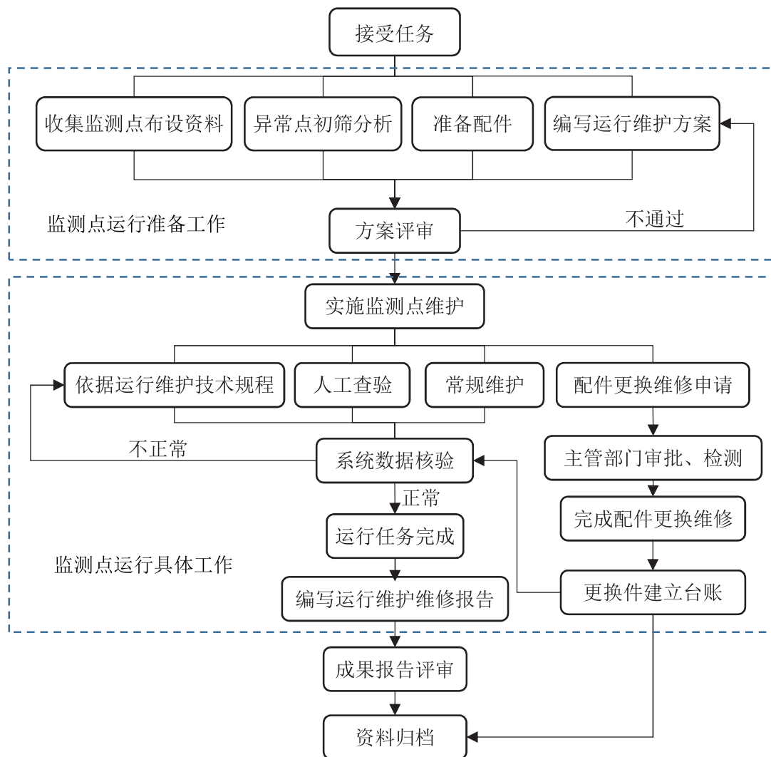
图2 监测点运行流程图
